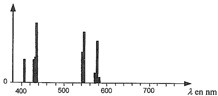
Figure 3 : lampe à vapeur de mercure
